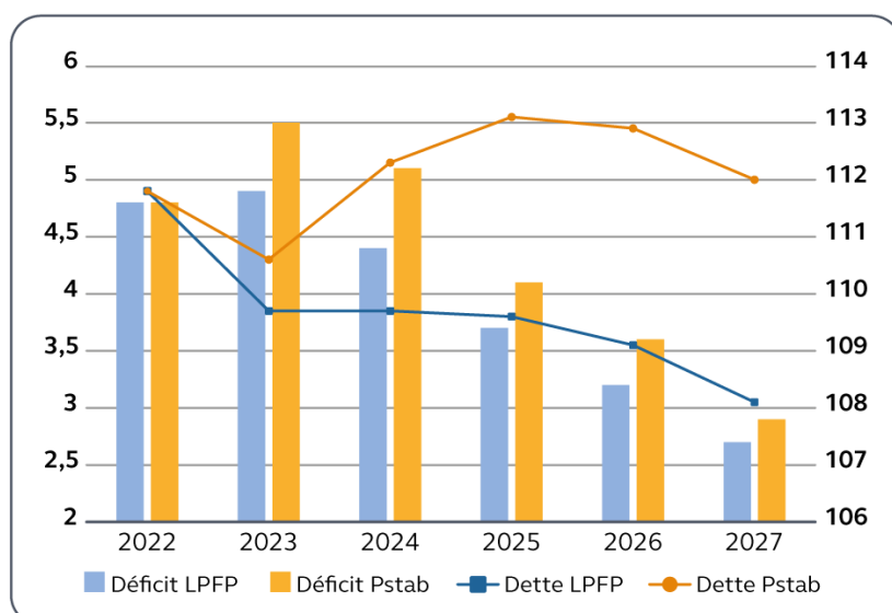
Graphique n° 19 : trajectoire du déficit public et de la dette publique (échelle de droite), en points de PIB
