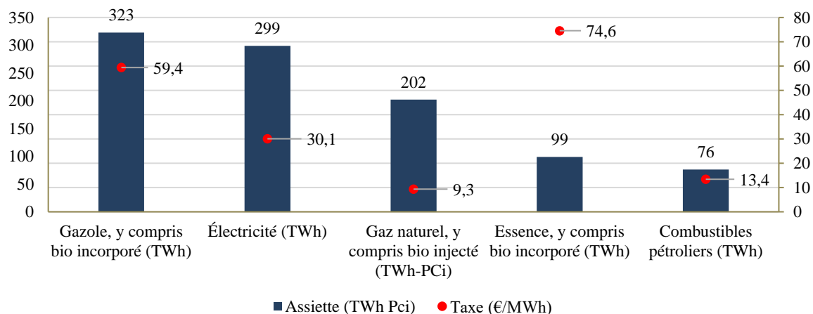
Graphique 13 : Niveau de taxation effective des différentes sources d'énergies
