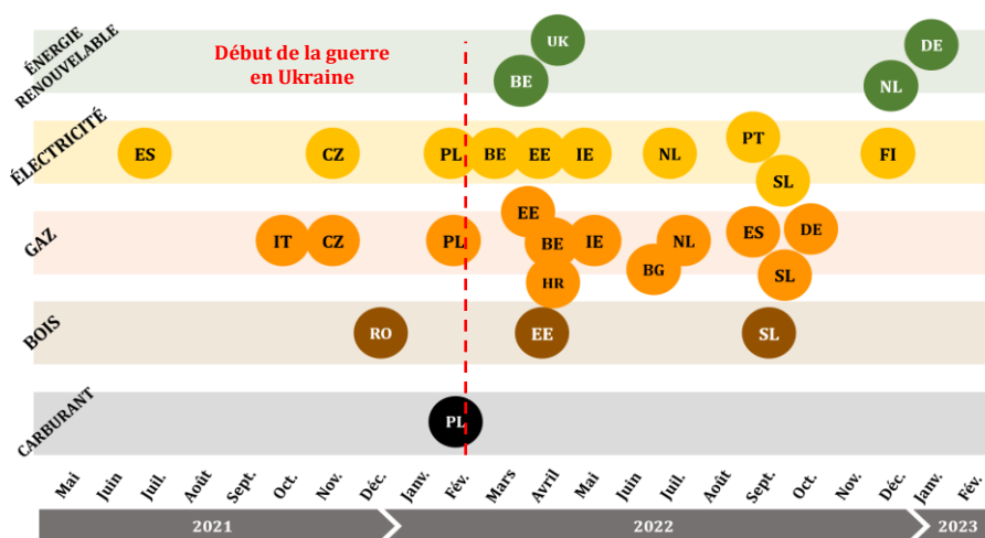
Figure 1 : Mesures de réduction de TVA dans le secteur de l'énergie dans l'UE à 28
